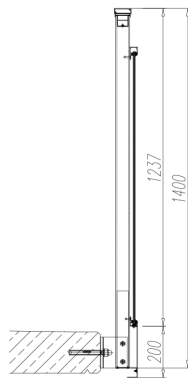
Balustrada FS-1
