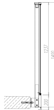
Balustrada FB-1
